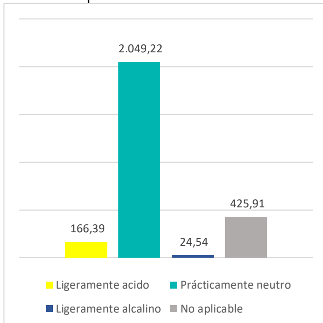
Gráfico 16. pH del suelo
