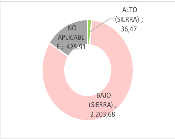
Gráfico 15. Materia orgánica del suelo
