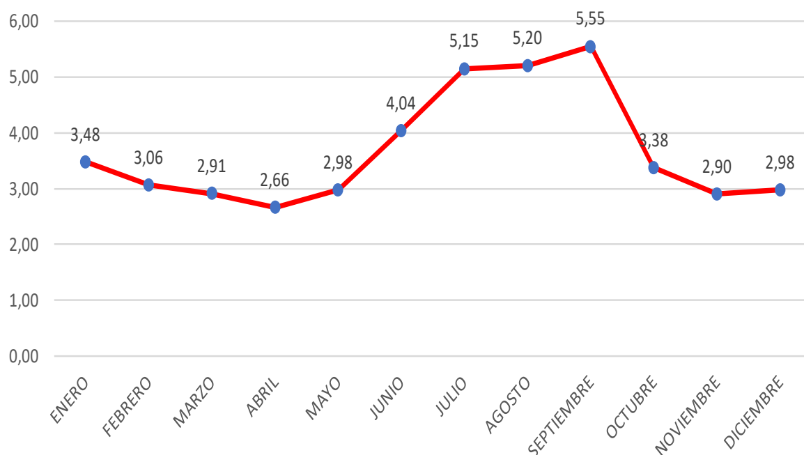
Gráfico 9. Velocidad mensual promedio del viento
