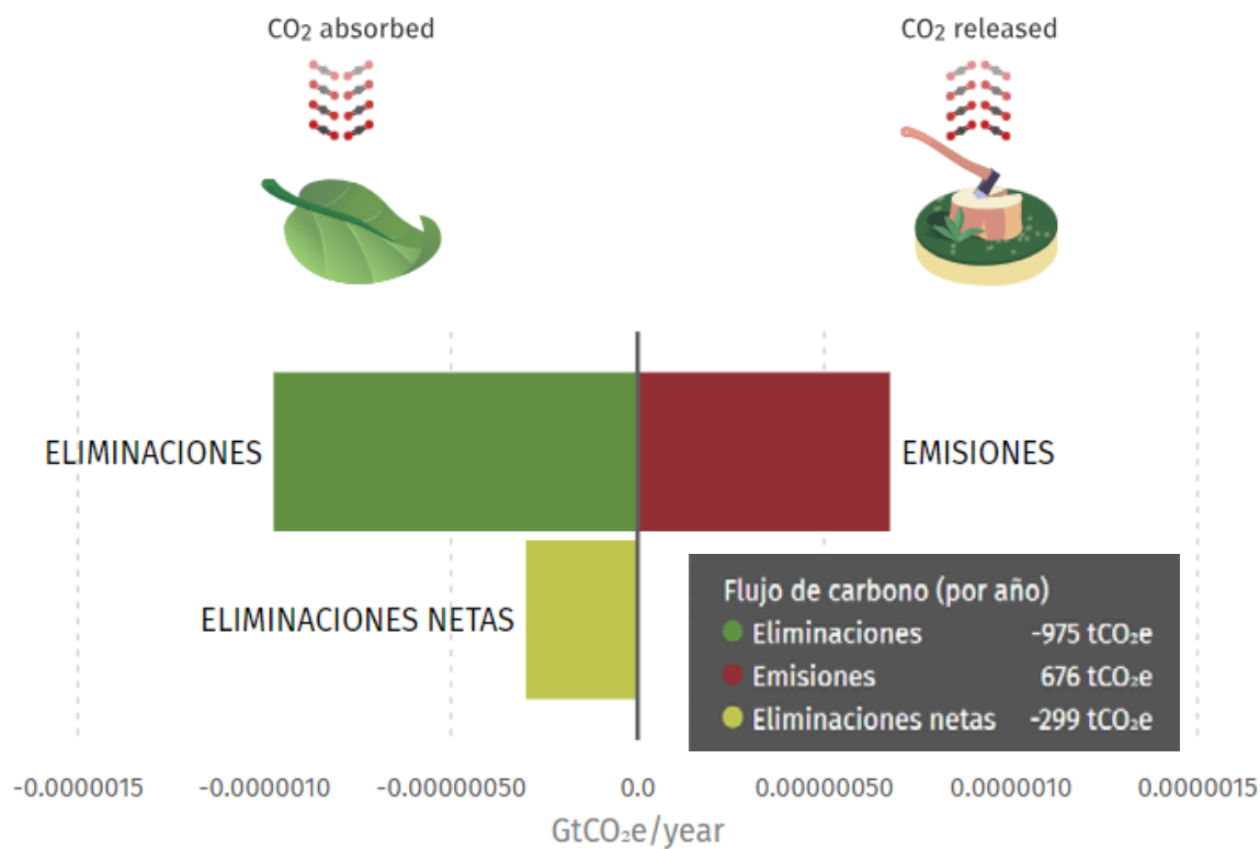
Imagen 2. Captura neta de Dióxido de carbono
