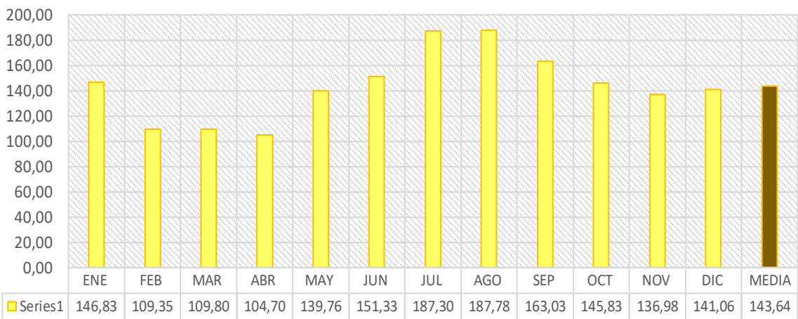
Gráfico 8. Horas de brillo solar mensual promedio
