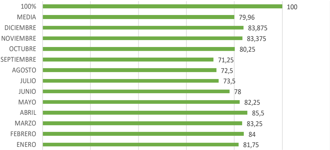
Gráfico 7. Régimen de humedad mensual
