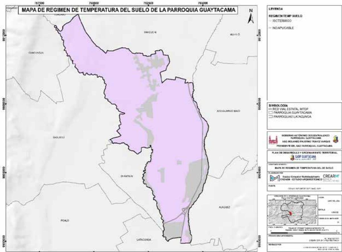
Mapa 16. Régimen de temperatura del suelo
