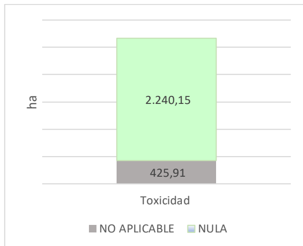
Gráfico 17. Toxicidad del suelo
