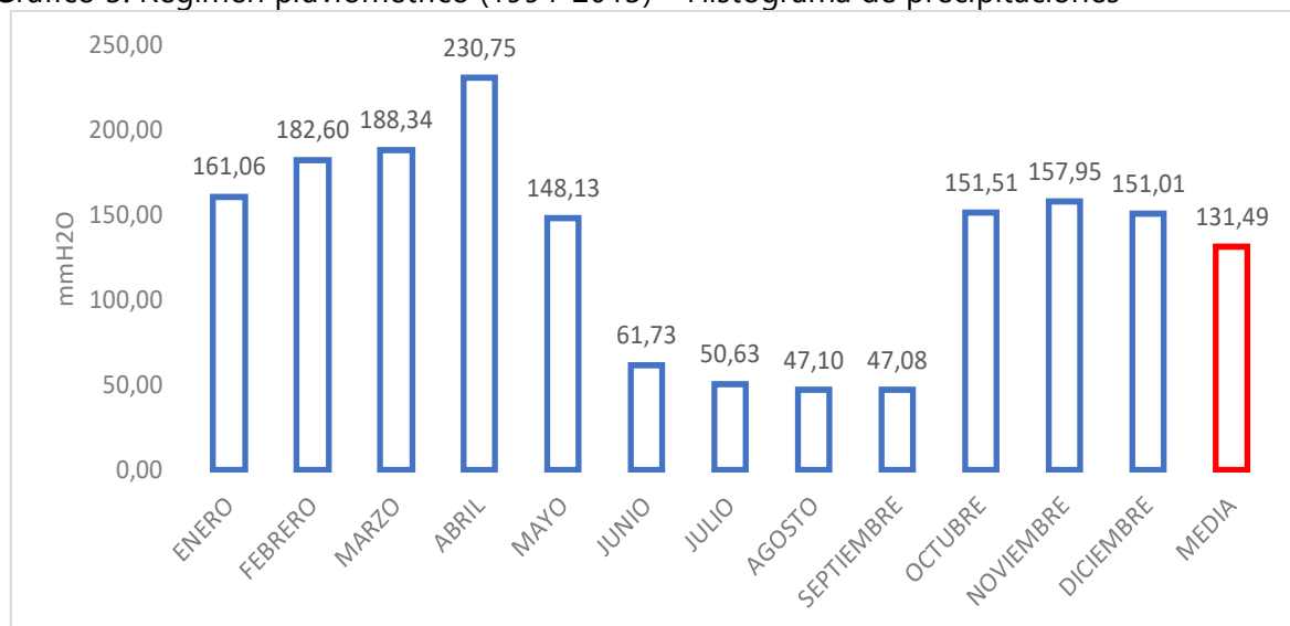
Gráfico 3. Régimen pluviométrico (1994-2013) – Histograma de precipitaciones
