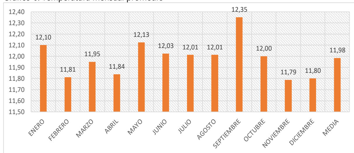
Gráfico 6. Temperatura mensual promedio
